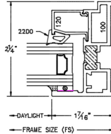
JAMB (no leg frame)
